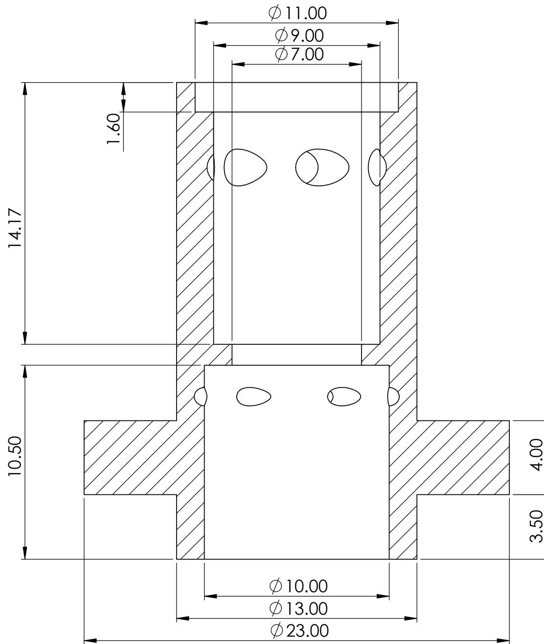
SECTION A-A
